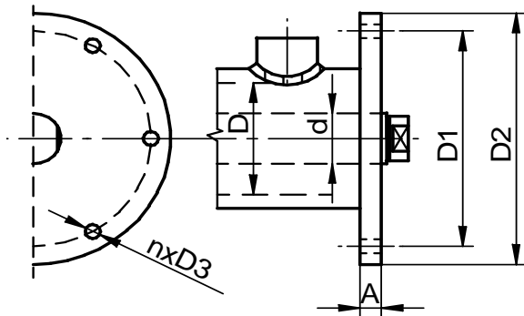
Príruba privarená na telo valca Prev. 3
